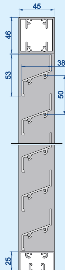
Vertikalschnitt: Maßstab 1:3
